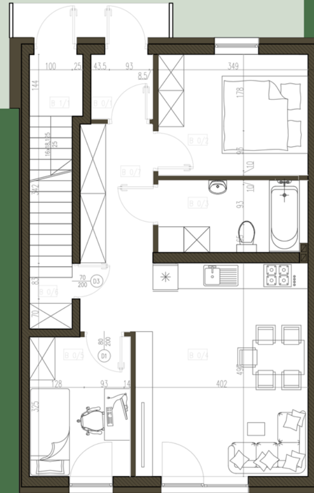
BUDYNEK D, LOKAL I 55,31 m 2
