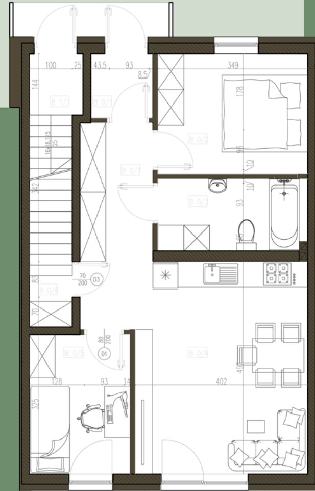
BUDYNEK B, LOKAL I 55,31 m 2
